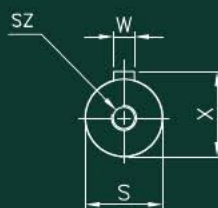
出力軸 OUTPUT SHAFT VIEW
