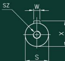
出力軸 OUTPUT SHAFT VIEW
