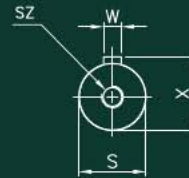
出力軸 OUTPUT SHAFT VIEW
