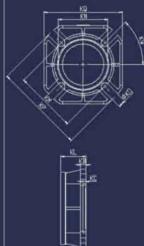
出力法蘭 OUTPUT-FLANGE
