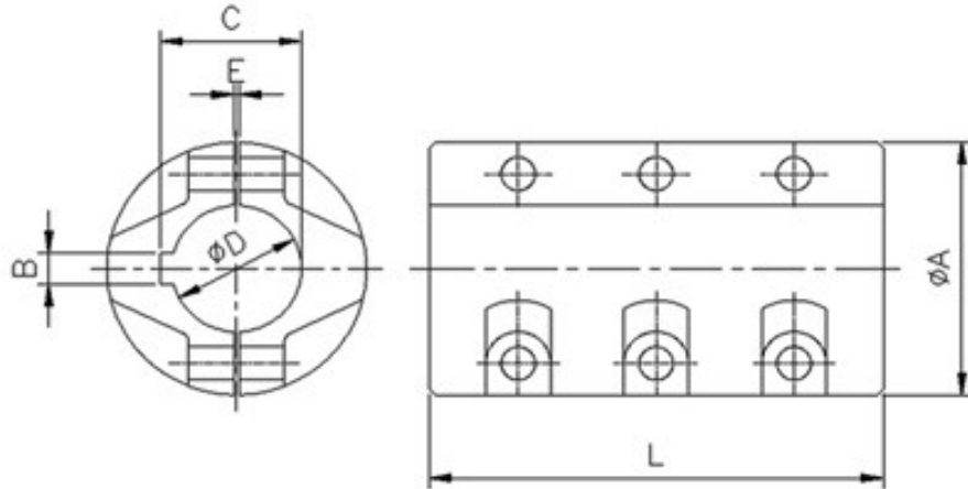
尺寸表
